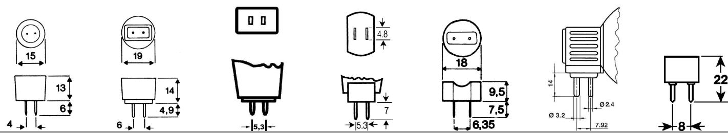
GZ4 GX5,3 GY5,3 G5,3/4,8 GX6,35-GZ6,35 GX7,9 G8
