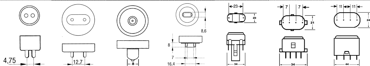
G5 G13 Fa8 R17d G23 2G7 2G11
