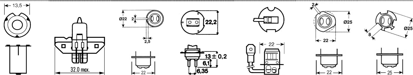
P13,5s PY16-1,25 P22D PG22 Pk22s P25d P25d4
